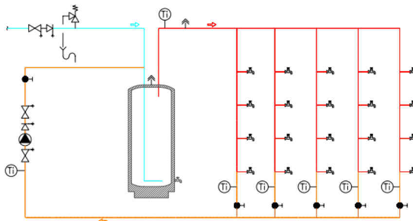
Figuur 1: Principeschets van een circulatieleiding met deelringen
